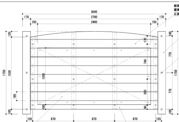
構造図
