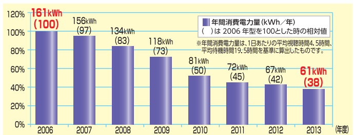
●テレビの年間消費電力量の推移 液晶テレビ 32V型
