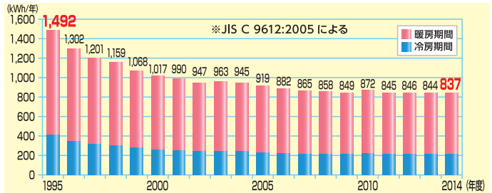
●エアコンの年間消費電力量の推移 ※購入状況はもっともよく使う機器についてお答えください。壁掛け型冷暖房兼用・冷房能力2.8kWクラス省エネ型代表機種種の単純平均値
